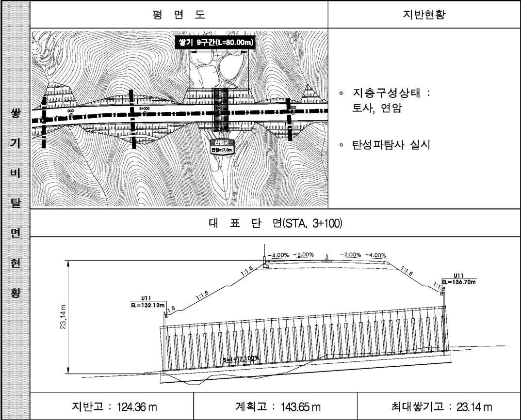
(9) 쌓기 9구간 (STA. 3+060~3+140, L=80.0m)
