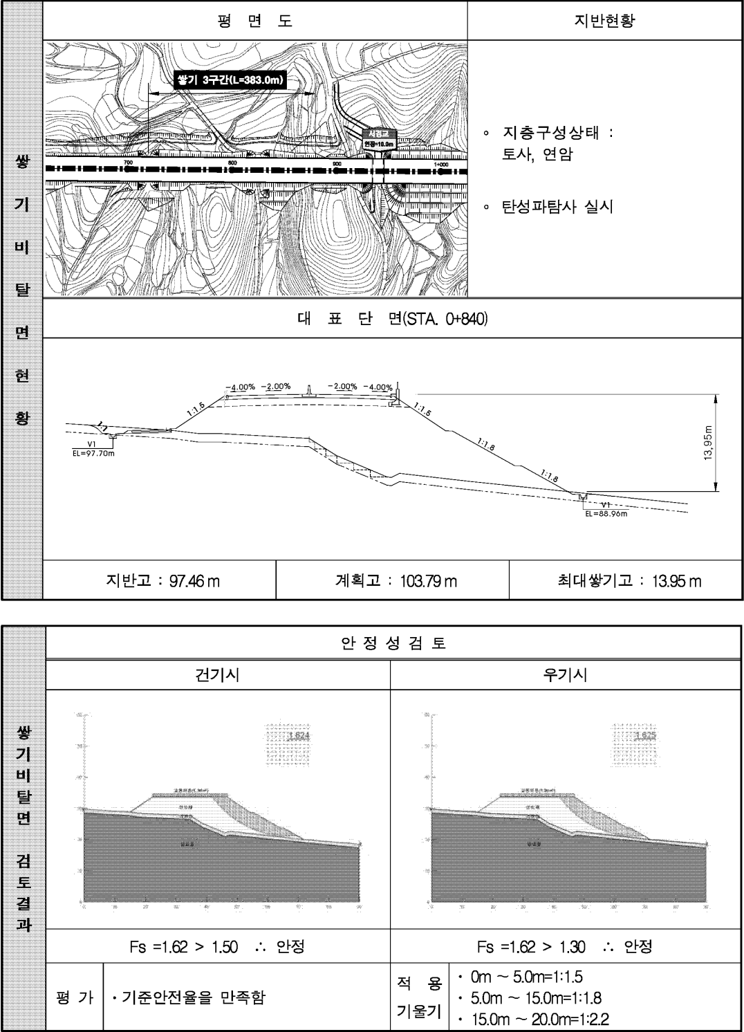
(3) 쌓기 3구간 (STA. 0+720~0+880, L=160.0m)
