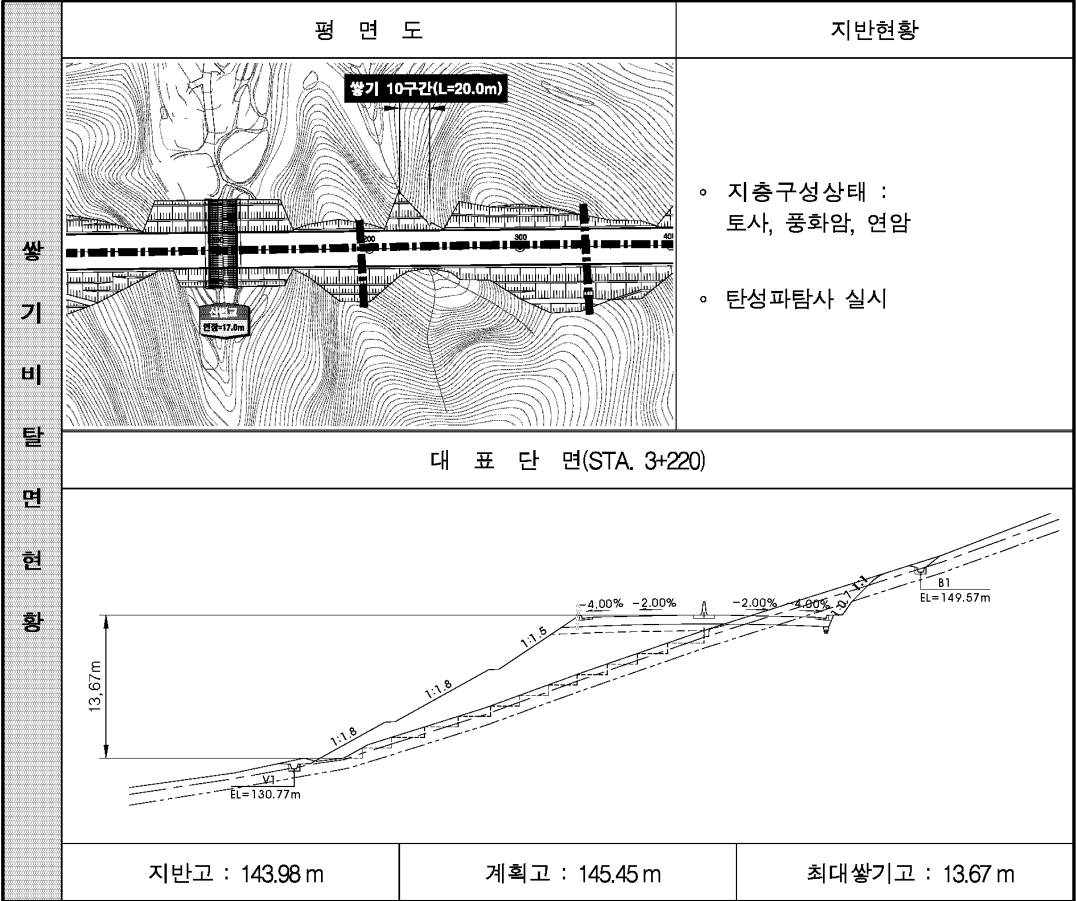
(10) 쌓기 10구간 (STA. 3+220~3+240, L=20.0m)
