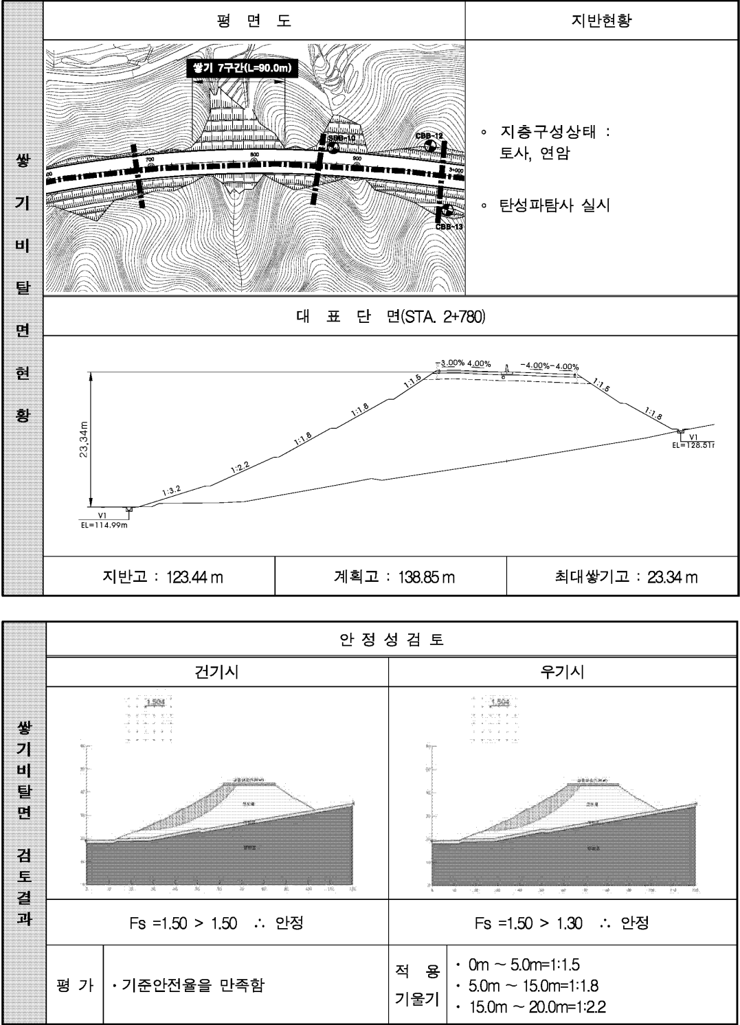
(7) 쌓기 7구간 (STA. 2+740~2+830, L=90.0m)
