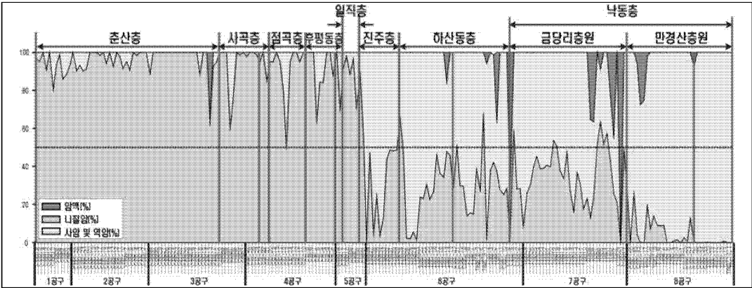
< 상주~영천고속도로 구간별 분포 총균 지질종단도>
