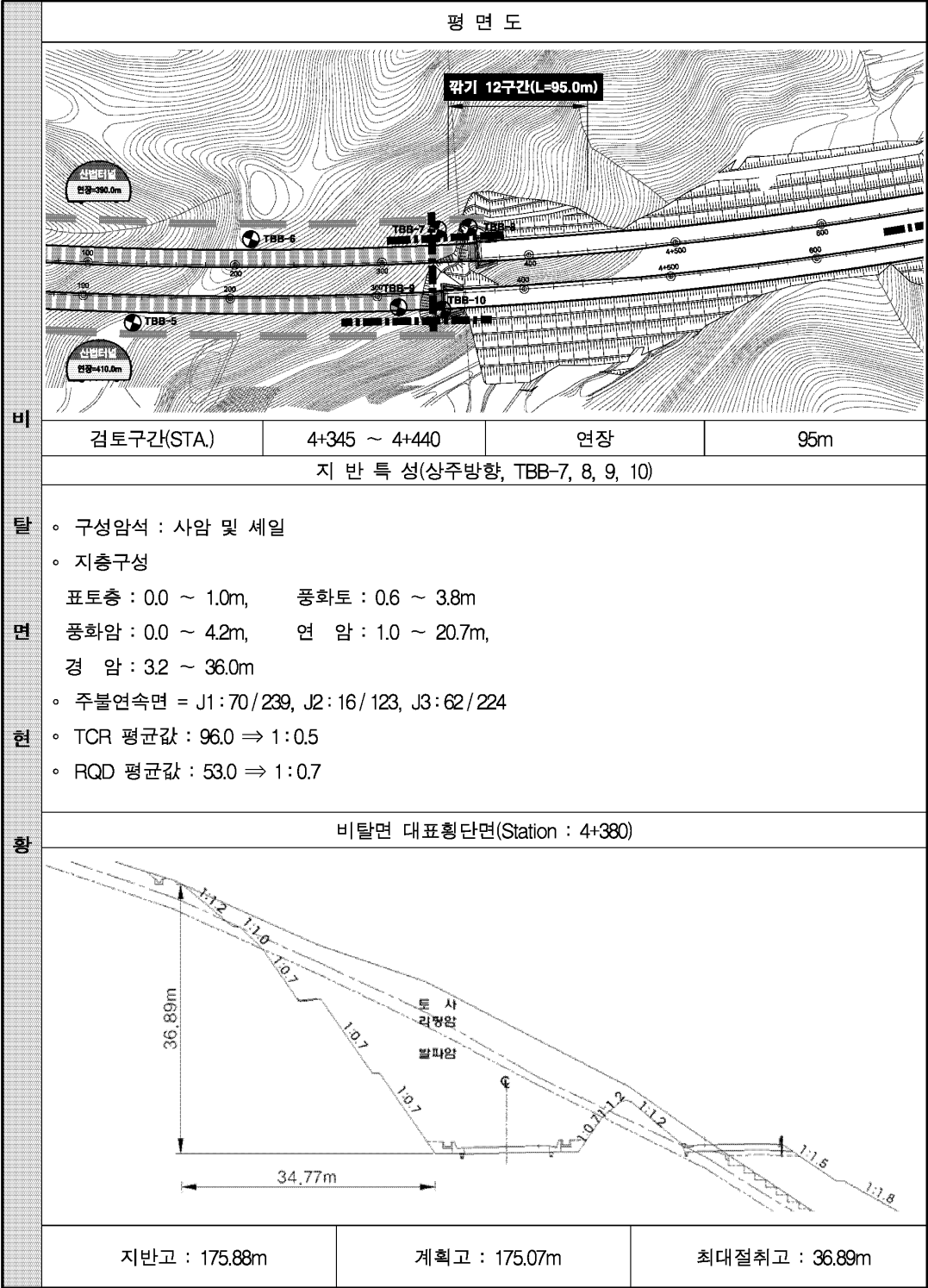
(12) 깎기 12구간(산법 T/L 종점부)
