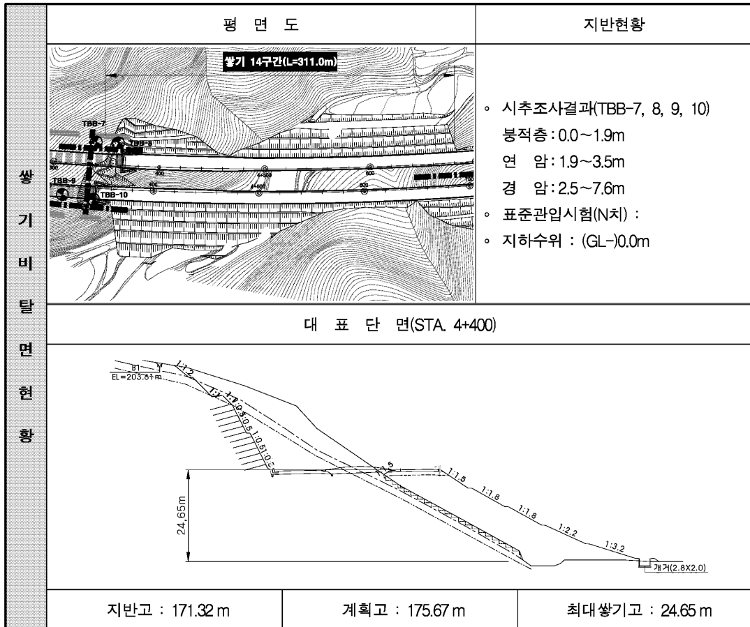
(14) 쌓기 14구간 (STA. 4+369~4+680, L=311.0m)
