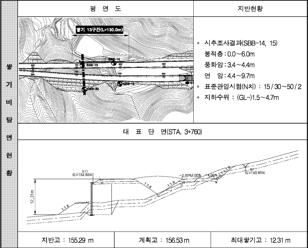
(13) 쌓기 13구간 (STA. 3+690~3+820, L=130.0m)
