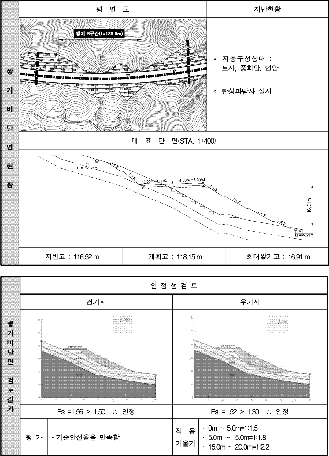
(5) 쌓기 5구간 (STA. 1+250~1+430, L=180.0m)
